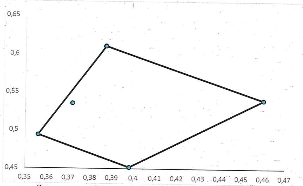
Допустимая область для желтого флуоресцентного цвета и фактические координаты цветности образца (куртка)
